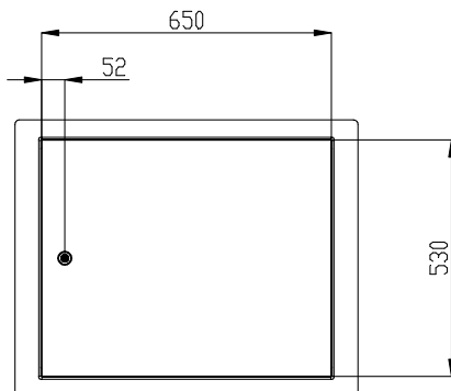
Boven aanzicht
